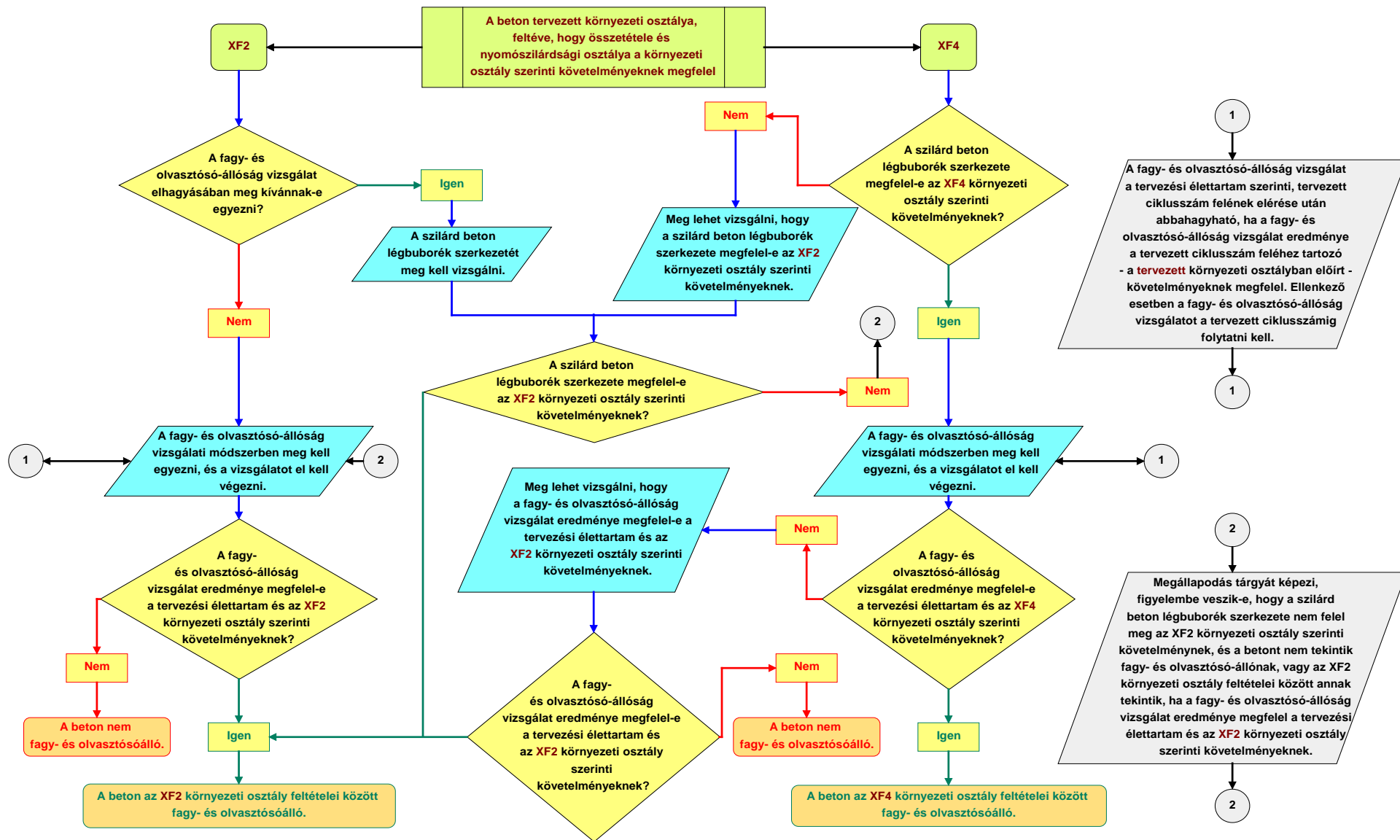
3. ábra: Légbuborékképző adalékszerrel készített, olvasztósó hatásának kitétt, 3%-os NaCl oldatban fagyasztott, XF2 és XF4 környezeti osztályú beton fagy- és olvasztósó-állóság vizsgálatának folyamatábrája
